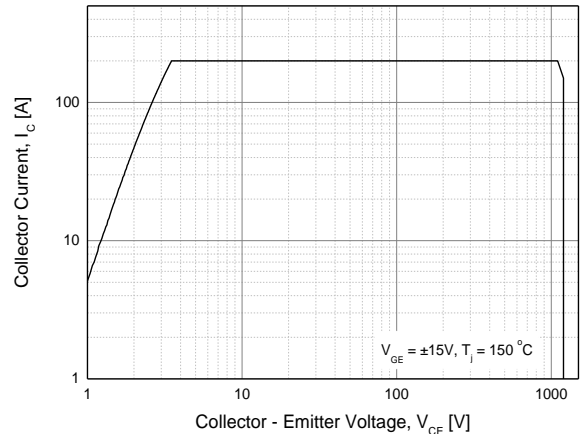
Fig. 12 RBSOA
