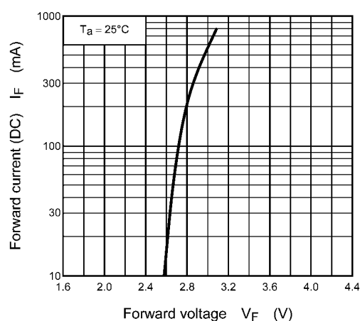
Fig. 8.1 I_F - V_F
